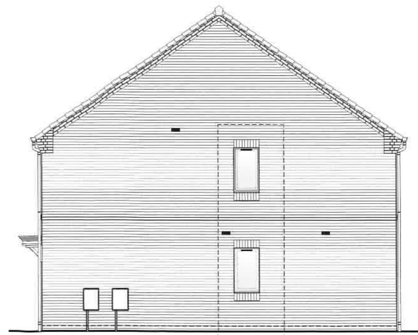
Right Elevation
